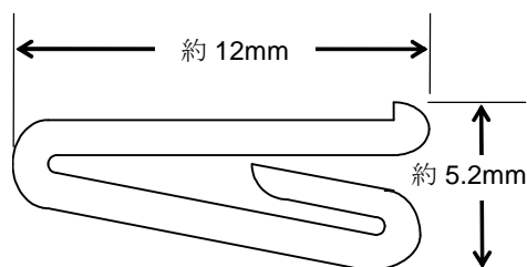
隠蔽ジョイナー断面形状
